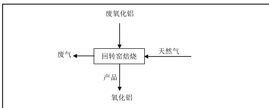
图 3.5-5 氧化铝产品生产工艺流程及产污环节示意图
