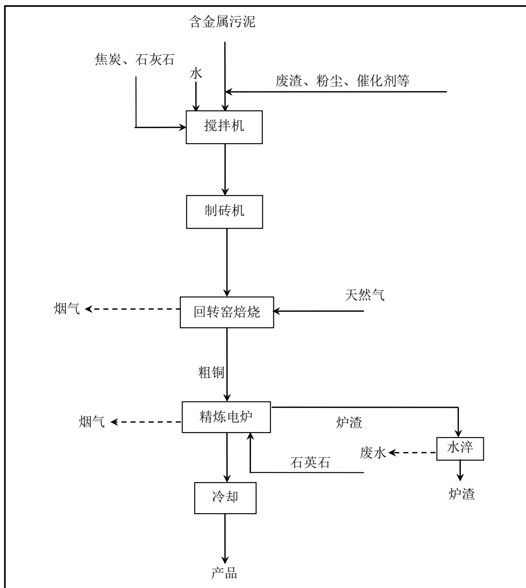
图 3.5-1 粗铜生产工艺流程及产污环节图
