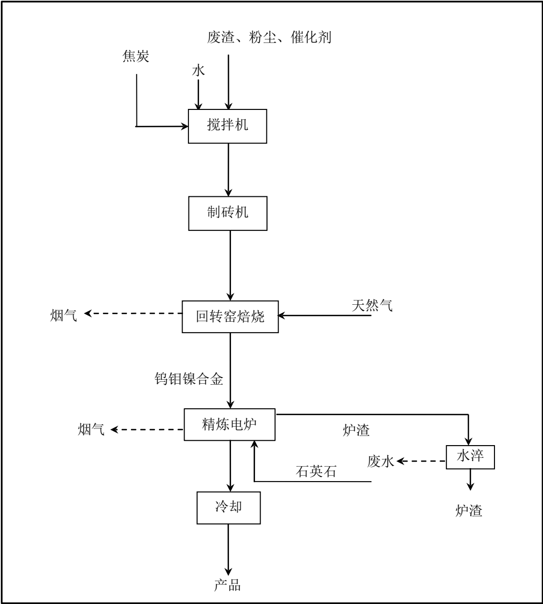
图 3.5-2 钨钼镍合金生产工艺流程及产污环节图
