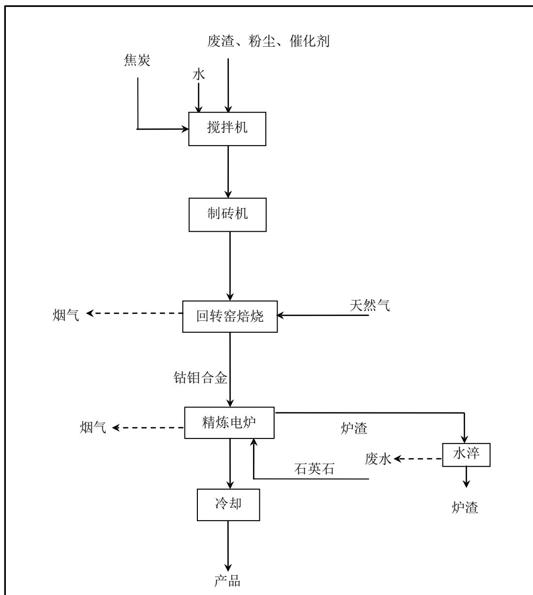
图 3.5-3 钴钼合金生产工艺流程及产污环节图
