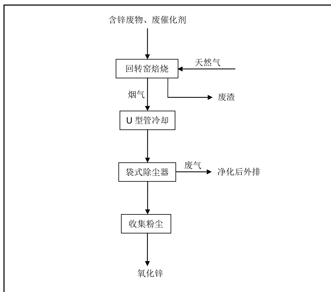
图 3.5-4 氧化锌产品生产工艺流程及产污环节示意图
